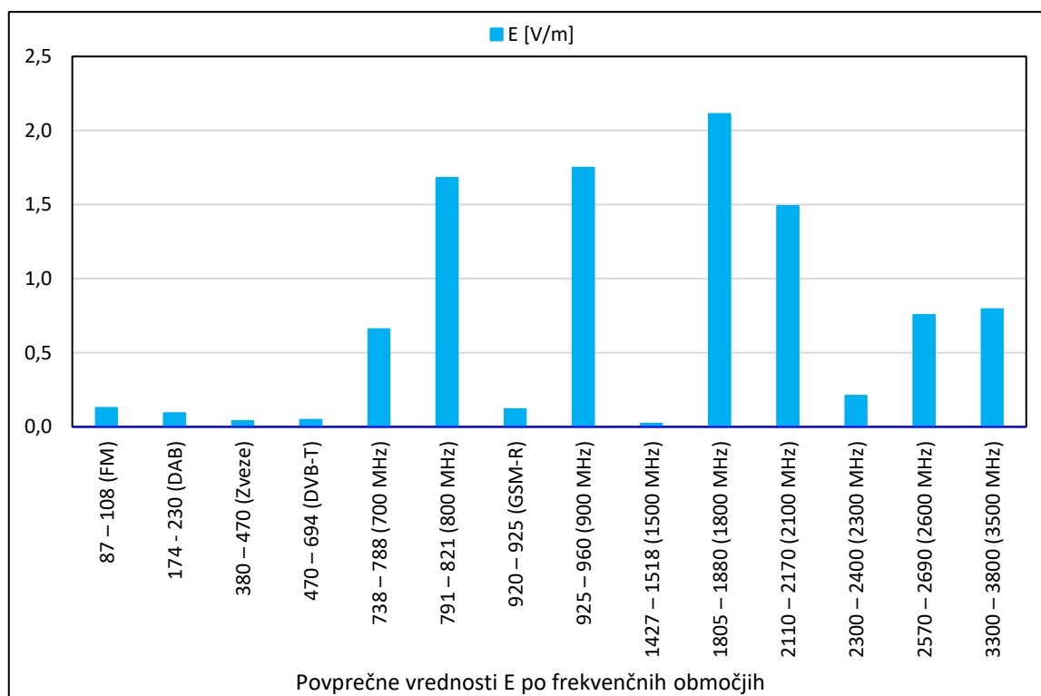
S 10: Povprečne vrednosti električnega polja po frekvenčnih pasovih.
